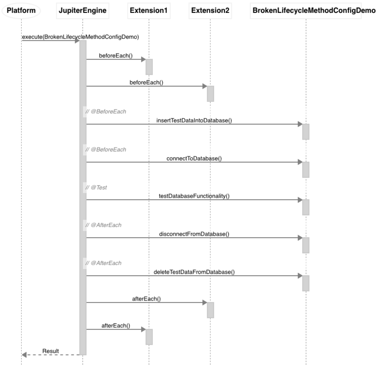
BrokenLifecycleMethodConfigDemo
